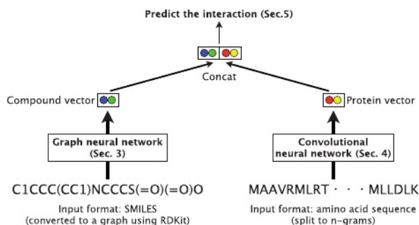
图 1. 所提出的 CPI 预测方法概述。化合物向量和蛋白质向量是通过图神经网络 (第 3 节) 和卷积神经网络 (第 4 节) 获得的低维实值表示，它们被连接起来并输入到分类器 (第 5 节) 中，以预测化合物和蛋白质是否相互作用。所提出的方法基于端到端表示学习，仅使用化合物和蛋白质的原始输入 (即 SMILES 和氨基酸序列)，而不是从数据库中提取的诸如分子指纹和蛋白质结构域之类的特征。更确切地说，我们分别将使用 RDKit 预处理的 SMILES 获得的分子图和基于 n-gram 氨基酸分割的蛋白质序列输入到 GNN 和 CNN 中。
